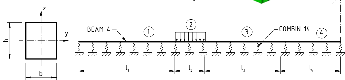
Prutový model betonového pražce B 91 S
