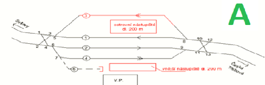
SCHEMA VARIANTY S VNĚJŠÍM NÁSTUPIŠTĚM
